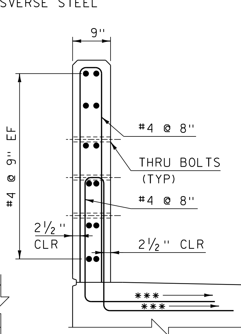
SECTION D-D
